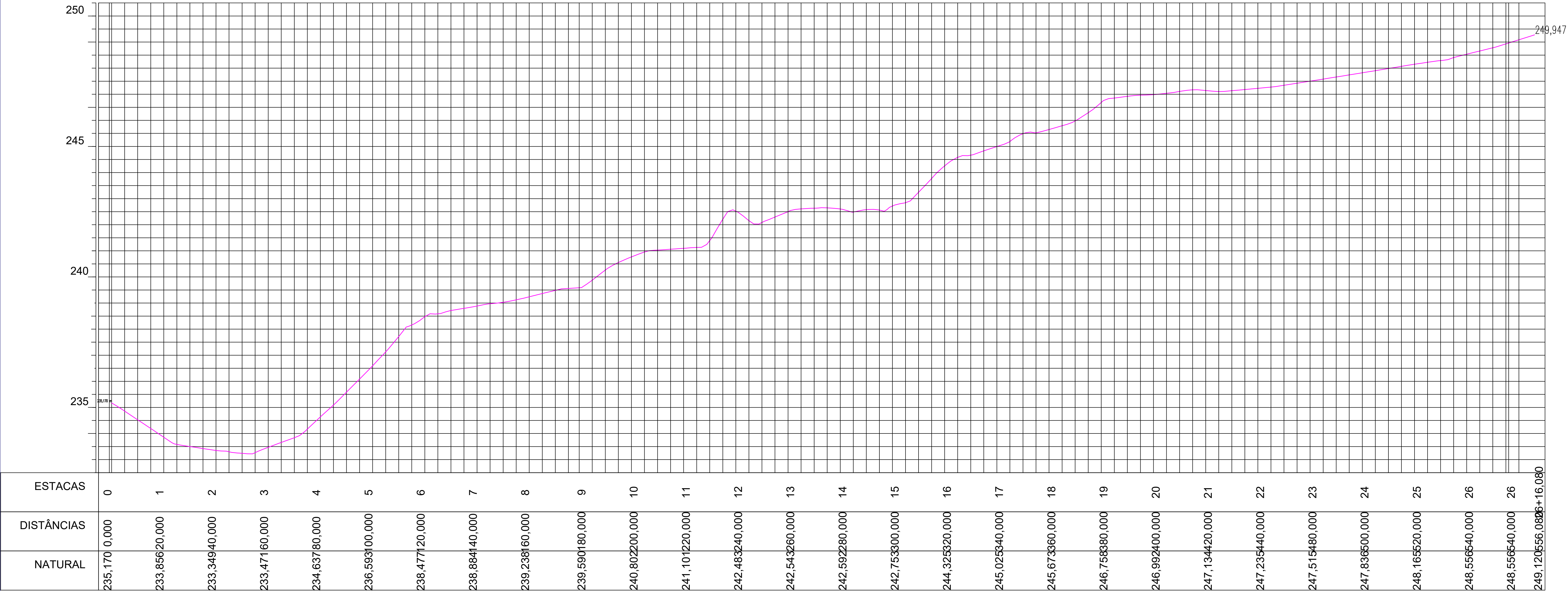
02 CORTE LONGITUDINAL
